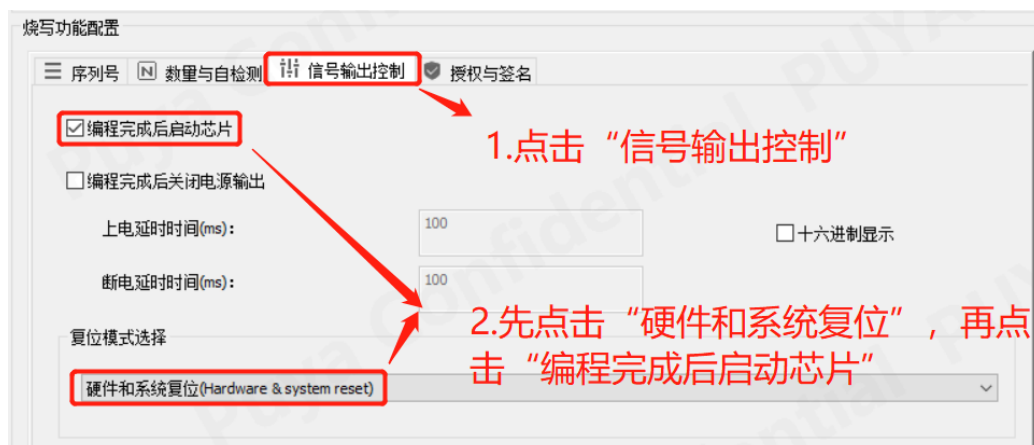
图 15-3 创芯工坊操作勾选“编程后重启芯片”
